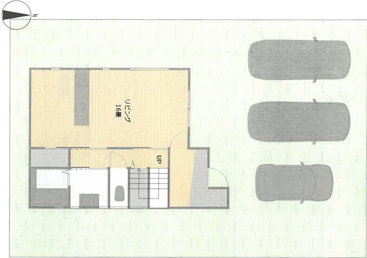
1階縮尺 1/100
